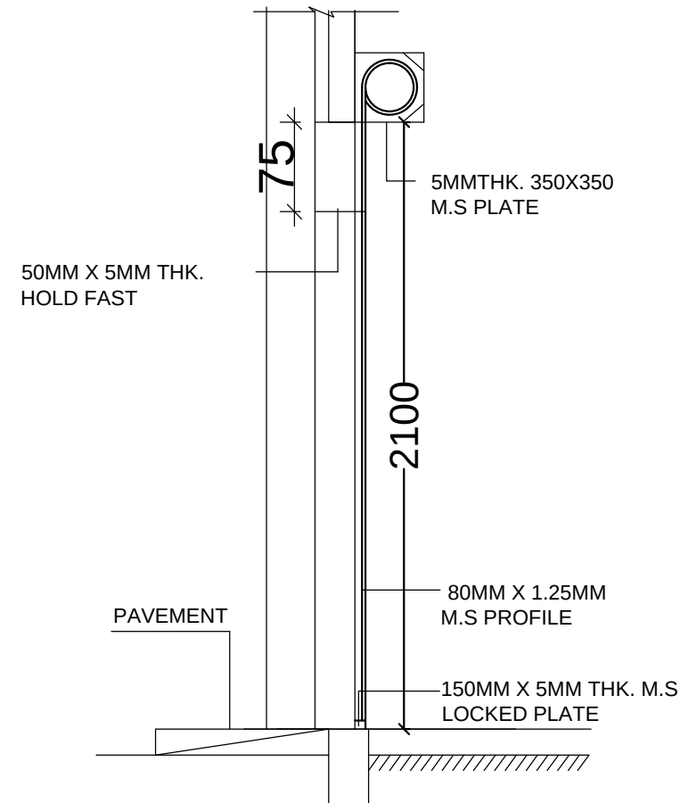
SECTION D-D
